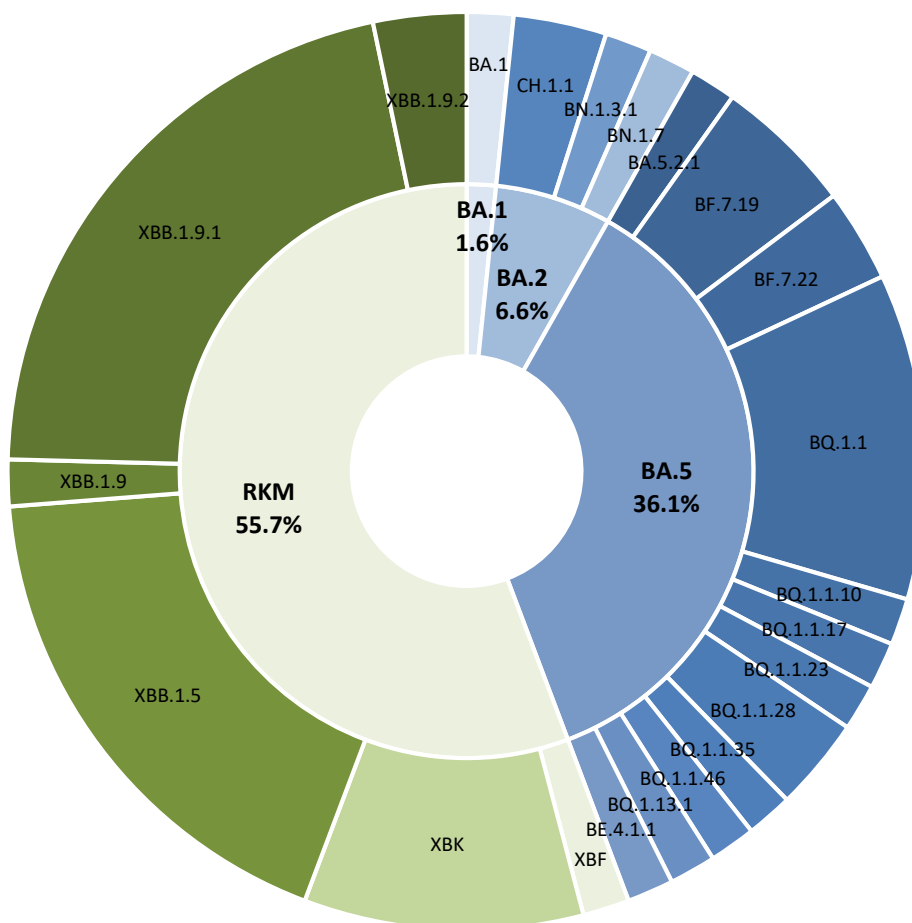
Slika 1. Razporeditev posameznih genetskih različic omikrona dokazanih v 8. tednu 2023. Zunanji obroč prikazuje posamezne dokazane različice z izpisom imena tistih, ki so bile prisotne v deležu > 1 %. Notranji obroč prikazuje starševsko linijo. Kategorija RKM predstavlja delež različic nastalih z rekombinacijo.
