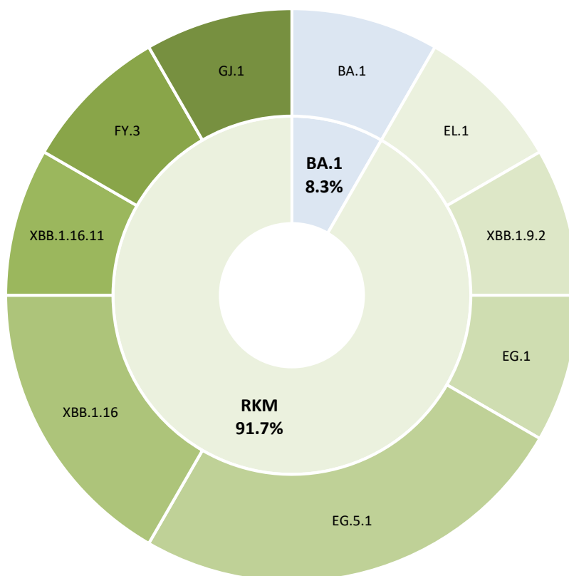
Slika 1. Razporeditev posameznih genetskih različic omikrona dokazanih v 30. in 31. tednu 2023. Zunanji obroč prikazuje posamezne dokazane različice z izpisom imena tistih, ki so bile prisotne v deležu \geq 1 %. Notranji obroč prikazuje starševsko linijo. Kategorija RKM predstavlja delež različic nastalih z rekombinacijo.
